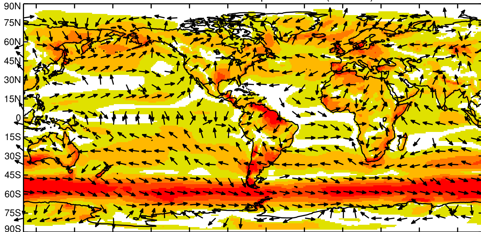
FAFMIP momentum flux perturbation ( 1e-3 Pa)
