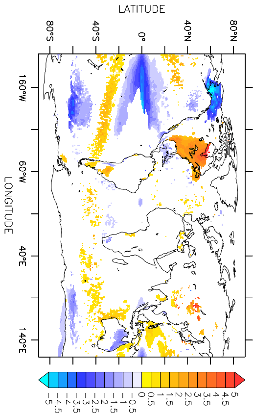
DJF TEMP | ROTVAR PC4
