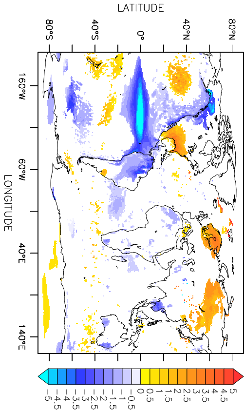
DJF TEMP | ROTVAR PC1
