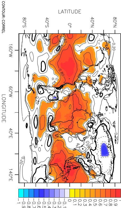
DEC EM [24]obs MSLP
