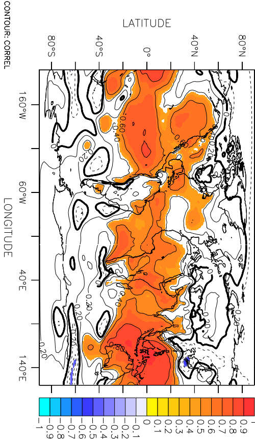
JAN EM [24]obs MSLP
