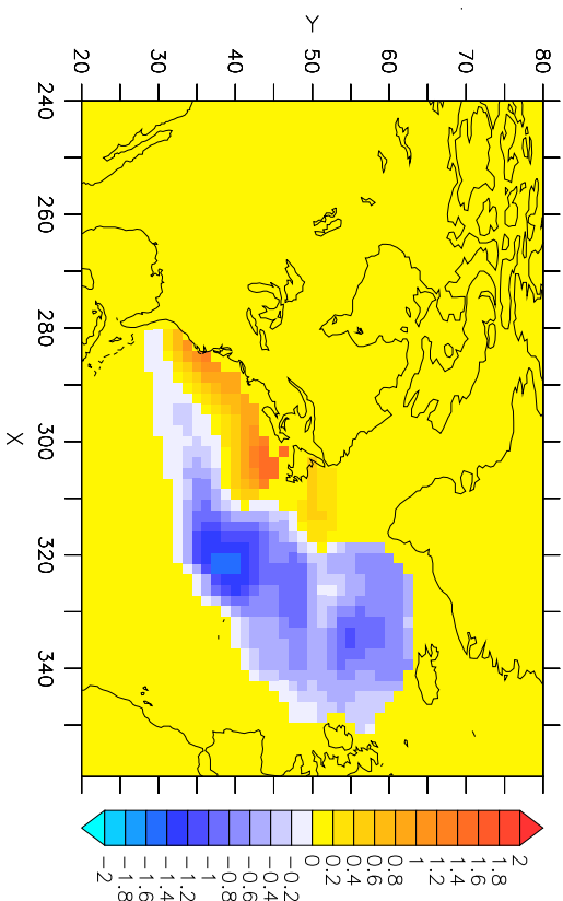
T:RAPIDSPG-CLIM
