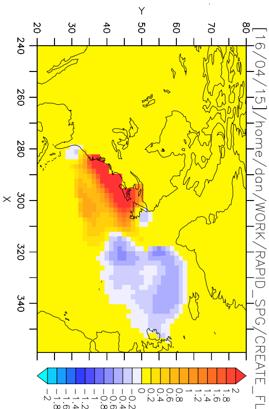
T:RAPIDSPG-CLIM
