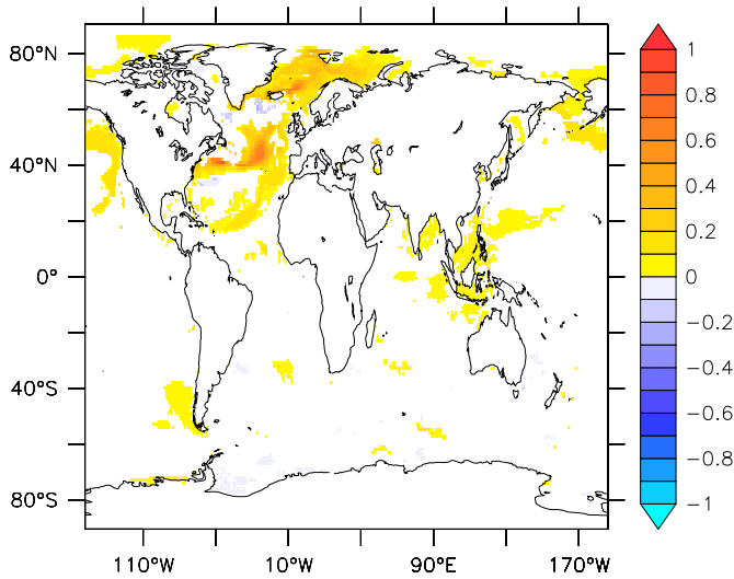
lag 0
