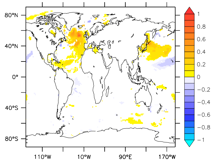
lag 6
