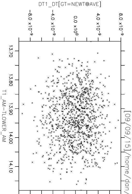
dTupper/dt vs Tupper-Tlower
